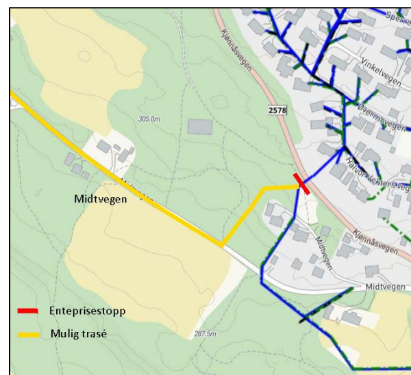
Figur 1. Kartutsnitt over eksisterende VA i prosjektområdet. Ny overføringsledning for vann skal gå etter Midtvegen, fra Grådalshaugen høydebasseng i vest, til tilknytning mot ledning fra Gunstadskogen høydebasseng i øst, med tilknytning rett ved Kjønnåsvegen Fv2578.
