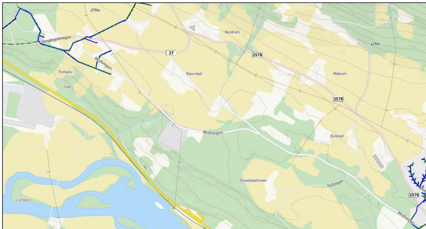
Figur 1. Kartutsnitt over eksisterende VA i prosjektområdet. Ny overføringsledning for vann skal gå etter Midtvegen, fra Grådalshaugen høydebasseng i vest, til tilknytning mot ledning fra Gunstadskogen høydebasseng i øst, med tilknytning rett ved Kjønnåsvegen Fv2578.
