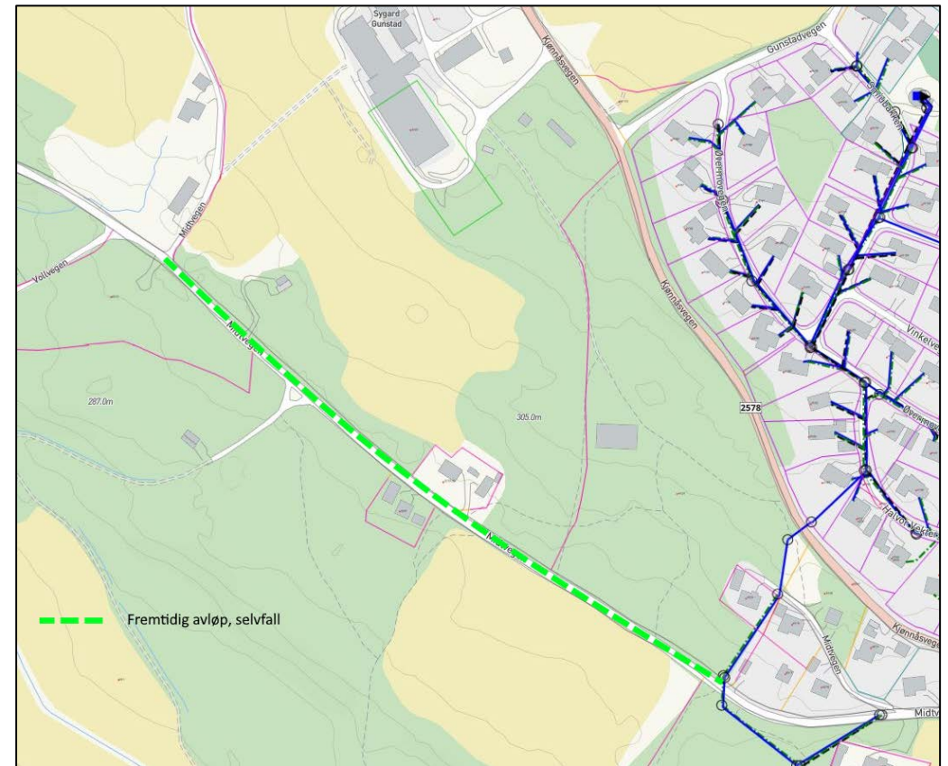
Figur 4. Østre ende av Midtvegen. Ny avløpsledning legges fra innkjøring til Nistugun Gunstad og østover til eksisterende kum ved Midtvegen 21.
