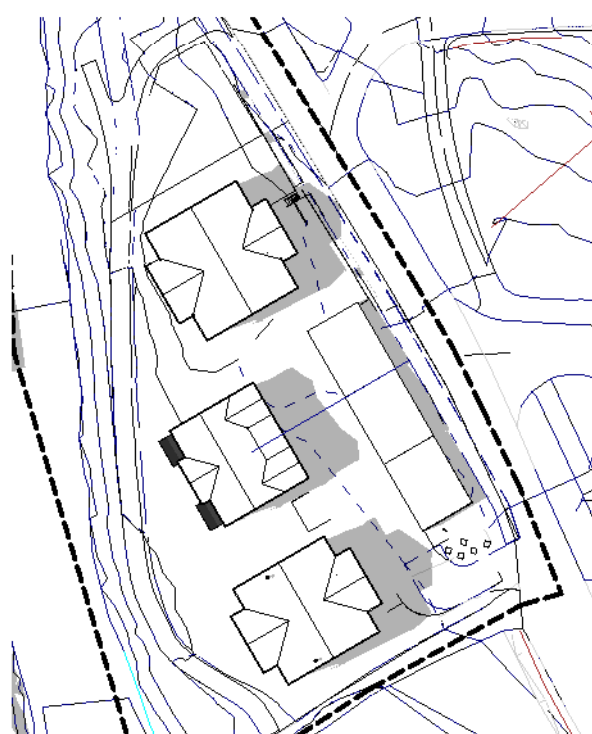
Solstudie 21.06 kl 15 1 : 1000
