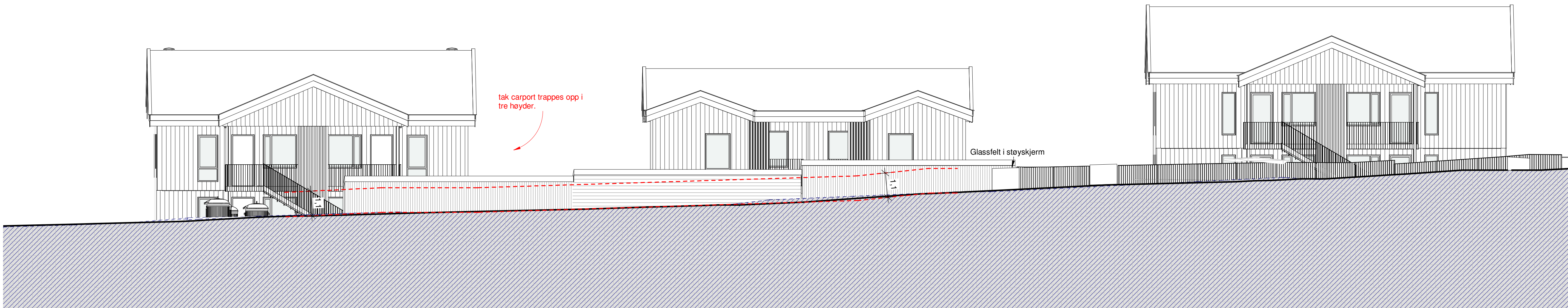
Snitt E 1 : 100
